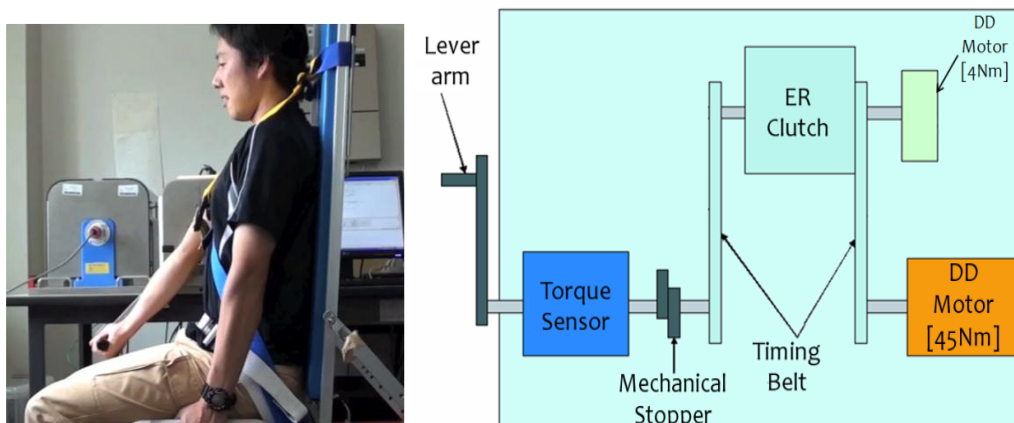
図 2-1. トレーニング装置の全体図および模式図
