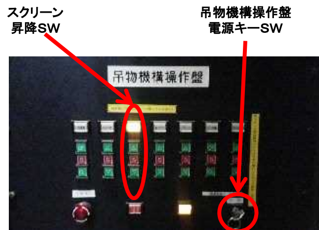
【吊物機構操作盤】
