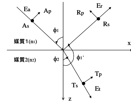
図 2.3 界面での反射と透過
