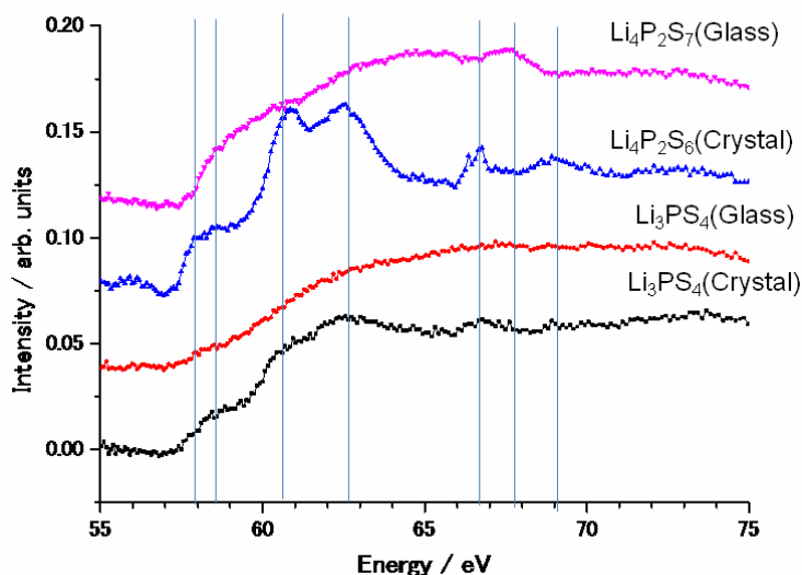
図 1. 標準試料の Li K-XANES 領域の比較 (試料電流測定法)。
