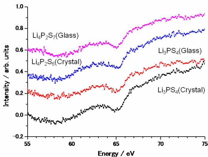
図 2. 標準試料の Li K-XANES 領域の比較 (全発光収量測定法)。
