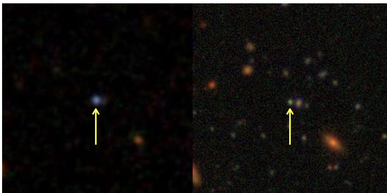
図 1: 本天体(黄色矢印)の SDSS 画像(左; 2002 年頃取得)とすばる望遠鏡 HSC 画像(右; 2018 年頃取得)。いずれも可視光のデータを用いた 3 色合成画像。HSC 画像の方が高感度なため、多くの暗い天体が検出されている。それら周りの天体と比較すると、本天体が大きな減光を示していることがわかる。
