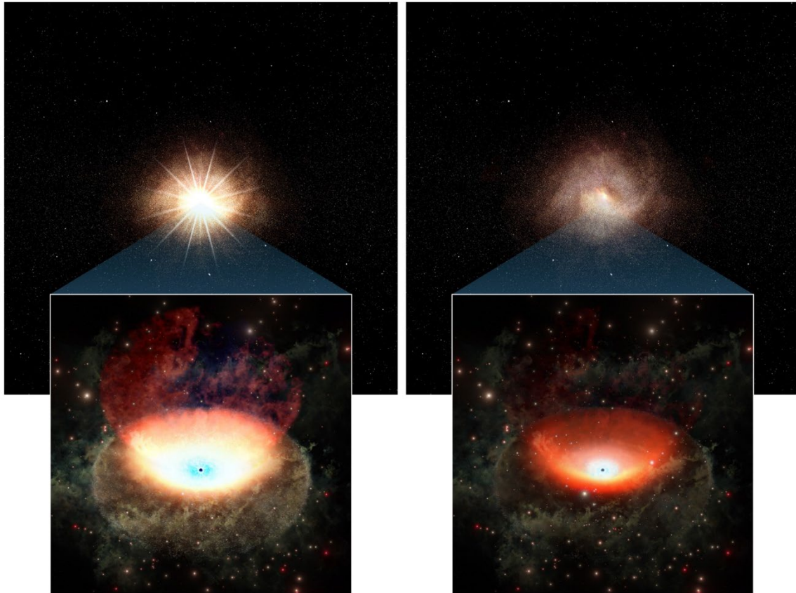
図 2: 明るい時期(左)と暗くなった時期(右)との天体の想像図の比較。上が銀河全体、下が中心部の超巨大ブラックホールまわりの拡大図。明るい時期は超巨大ブラックホール(中心部の黒い領域)周りの降着円盤(青白い部分)やその周辺のダスト等で構成されるトーラス状の構造が明るく輝いているのに対して、超巨大ブラックホールへのガス流入が少なくなると、全体が暗くなる。
