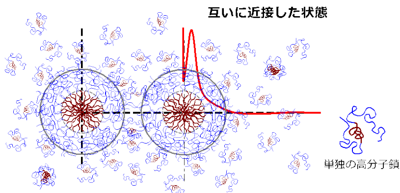
図4：本研究で初めて明らかとなった高分子ミセルや治療薬を包含した高分子ミセルの相互作用場(上図グラフ)
