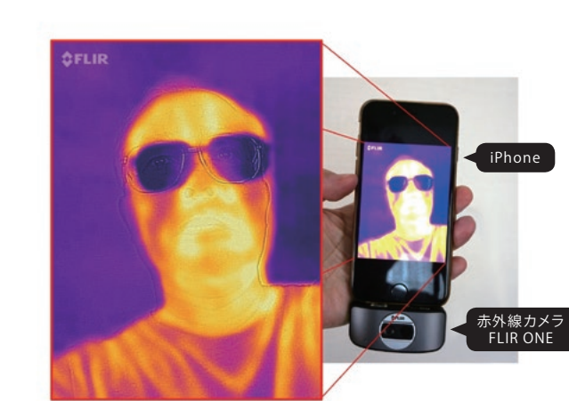
スマートフォン用赤外線カメラと赤外線画像
