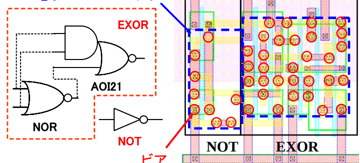
(a) 基本素子回路
