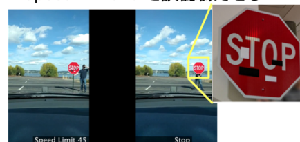
図 4. Adversarial Examples 攻撃
