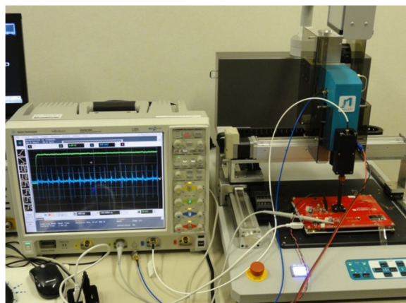
図 5. サイドチャネル攻撃評価環境
