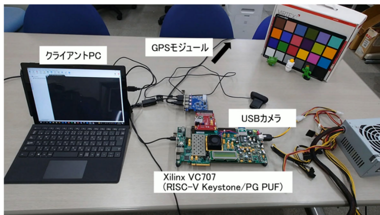
図 6. RISC-V (オープンコア CPU) を使った PUF デモシステム
